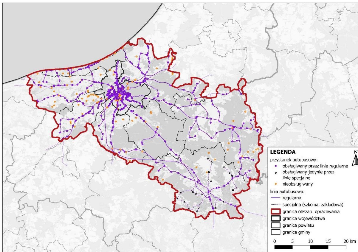
Rysunek 3 Sieć autobusowa przewoźników prywatnych
